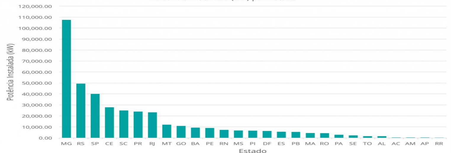
Potência Instalada (kW) por Estado
