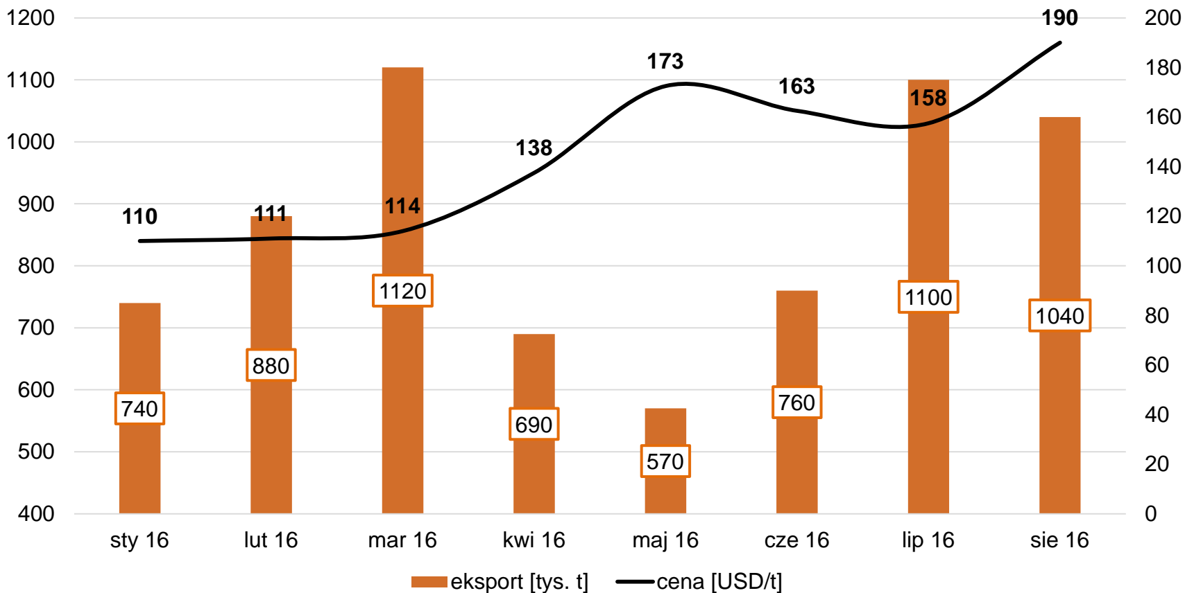
Rys. 21. Eksport i ceny koksu chińskiego w 2016 [ tys. ton, USD/t]
