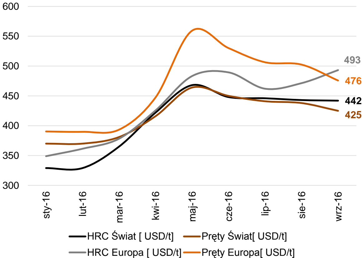
Rys. 4. Ceny stali na świecie w 2016 roku [USD/t]
