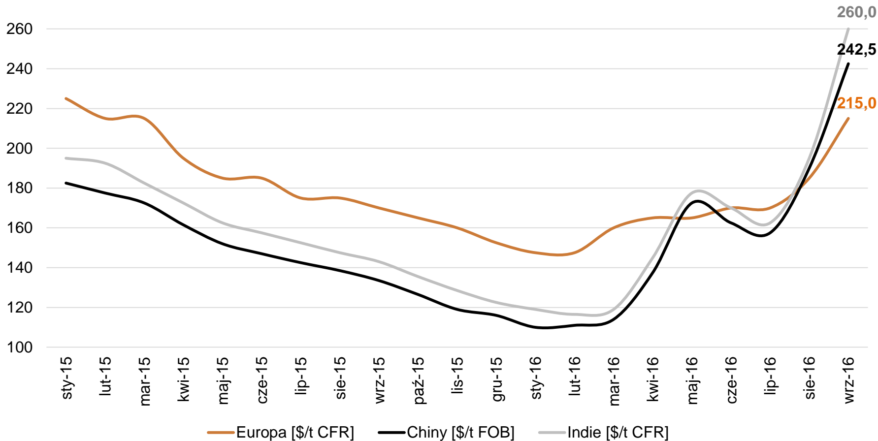
Rys. 24. Ceny koksu wielkopiecowego na światowych rynkach w latach 2015-2016 [USD/t]
